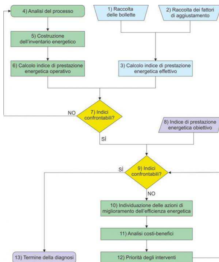
Figura 2 - Schema di flusso indicativo della Diagnosi Energetica
